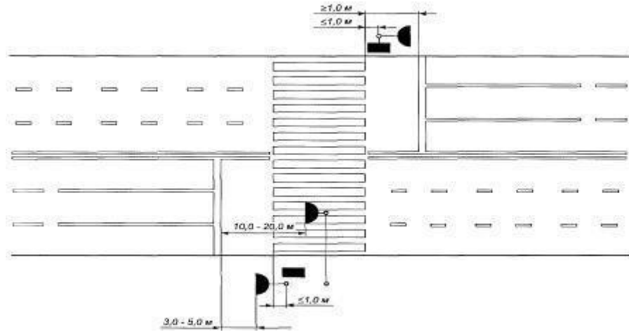
Рис. 5 Пример размещения светофор и нанесения разметки на регулируемом пешеходном переходе.
